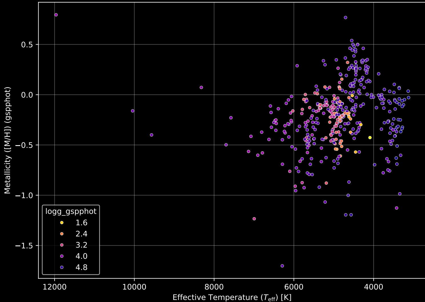
APOGEE DR17 Field: [120+45] Stellar Population Parameters (n= 420)
